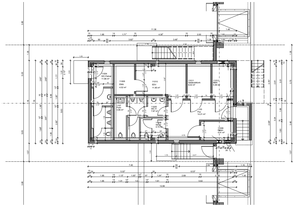
Grundriss EG Hallenbüro (B11) 1:50
