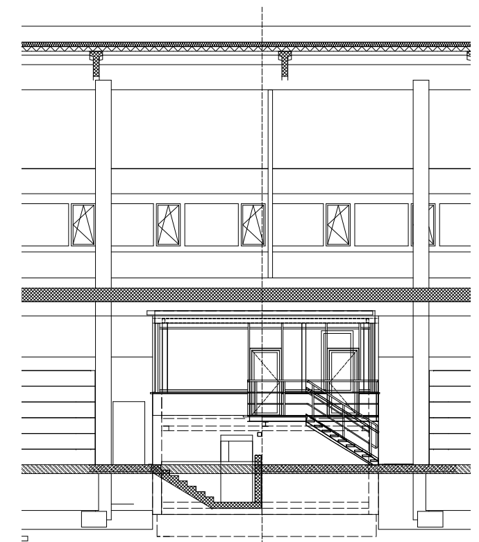
Ansicht Norden Hallenbüro 11
