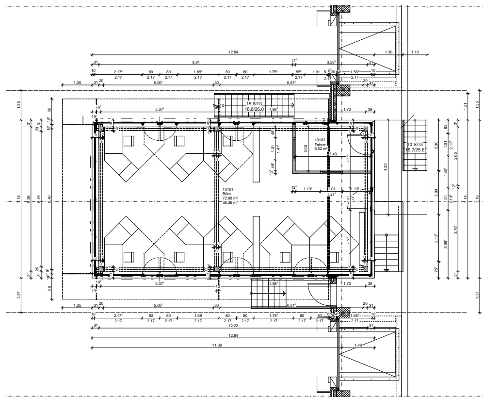
Grundriss OG Hallenbüro (B11) 1:50
