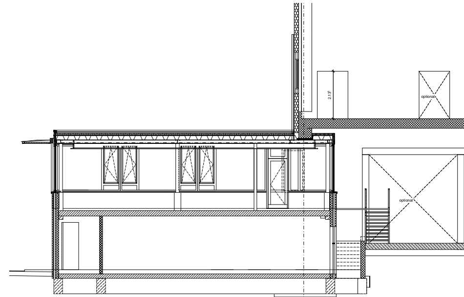
Schnitt 11.4 Hallenbüro 11
