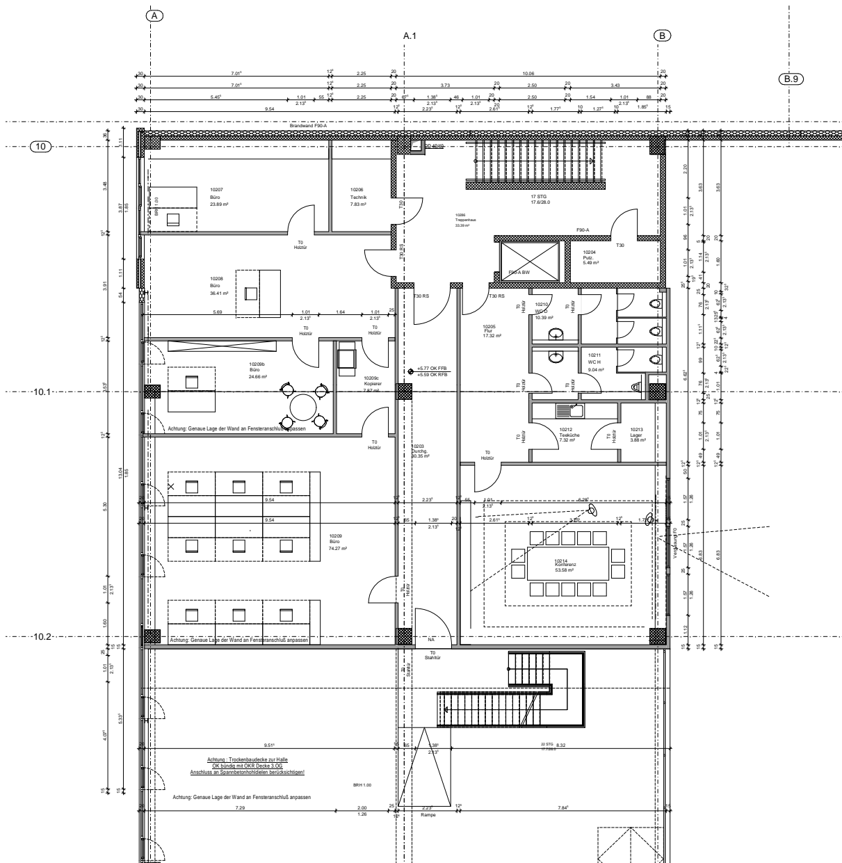
2. Obergeschoss
