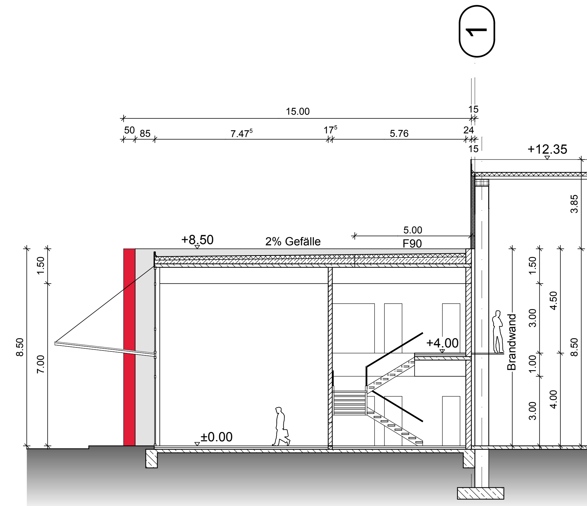
SCHNITT A-A
