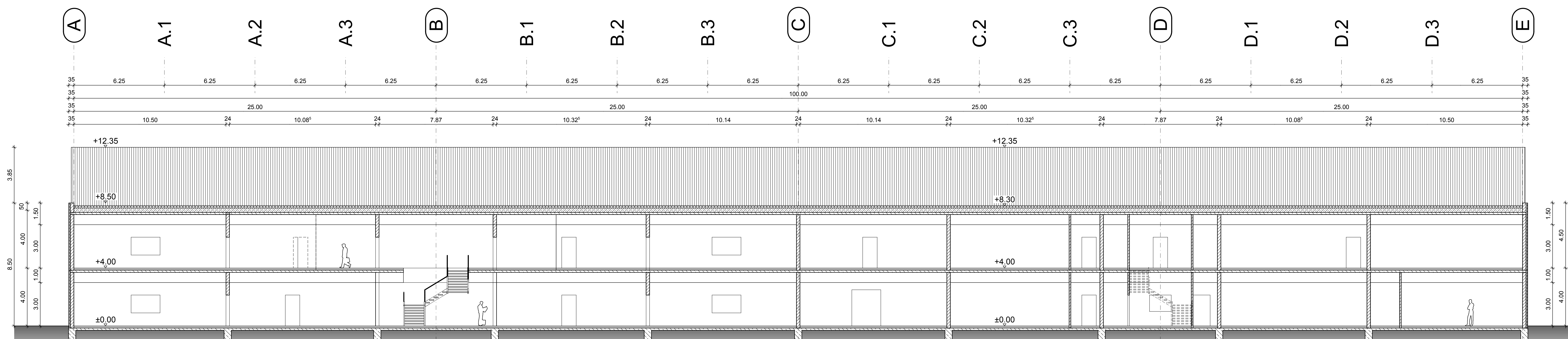
SCHNITT C-C
