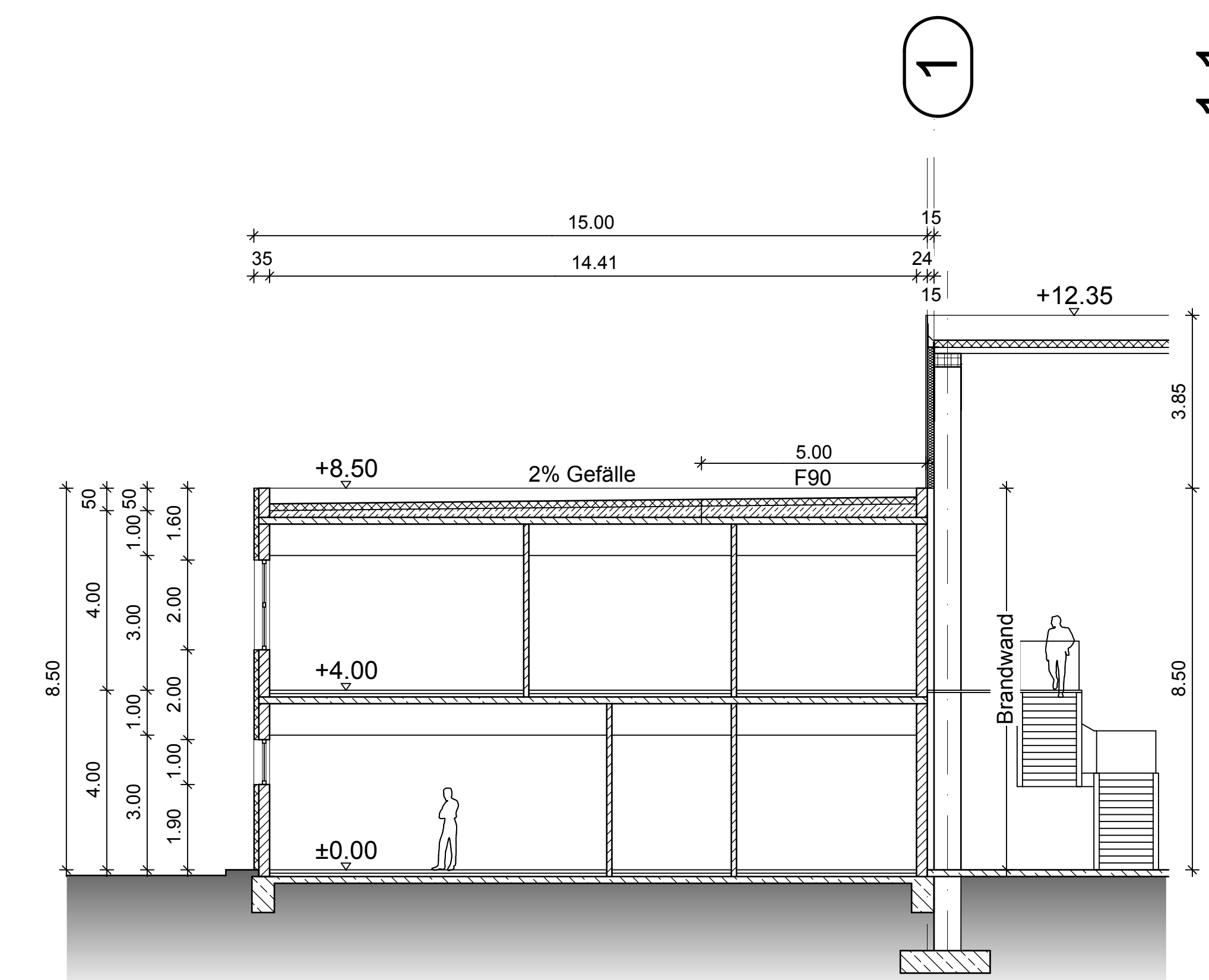
SCHNITT B-B
