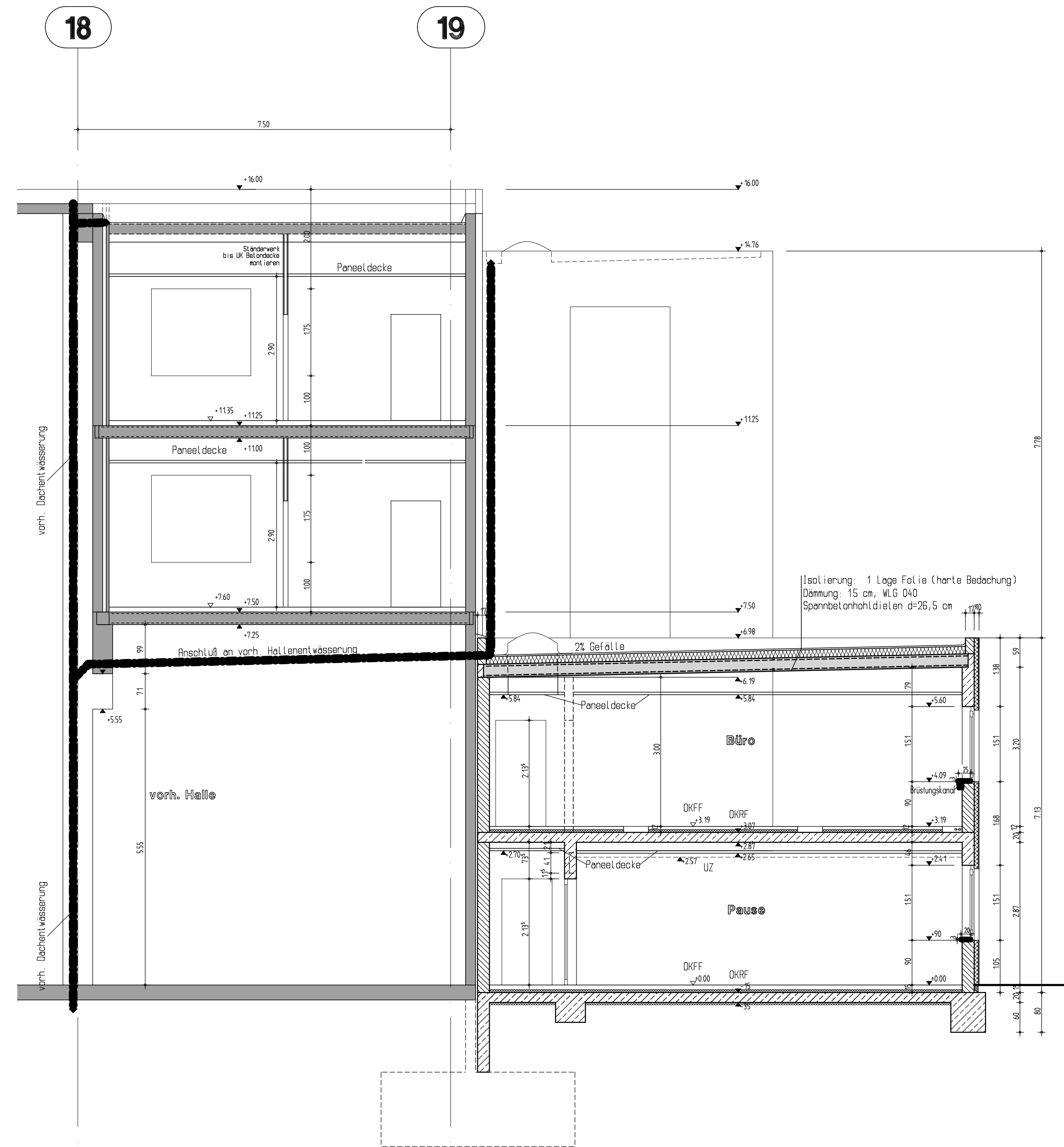
Schnitt 2-2
