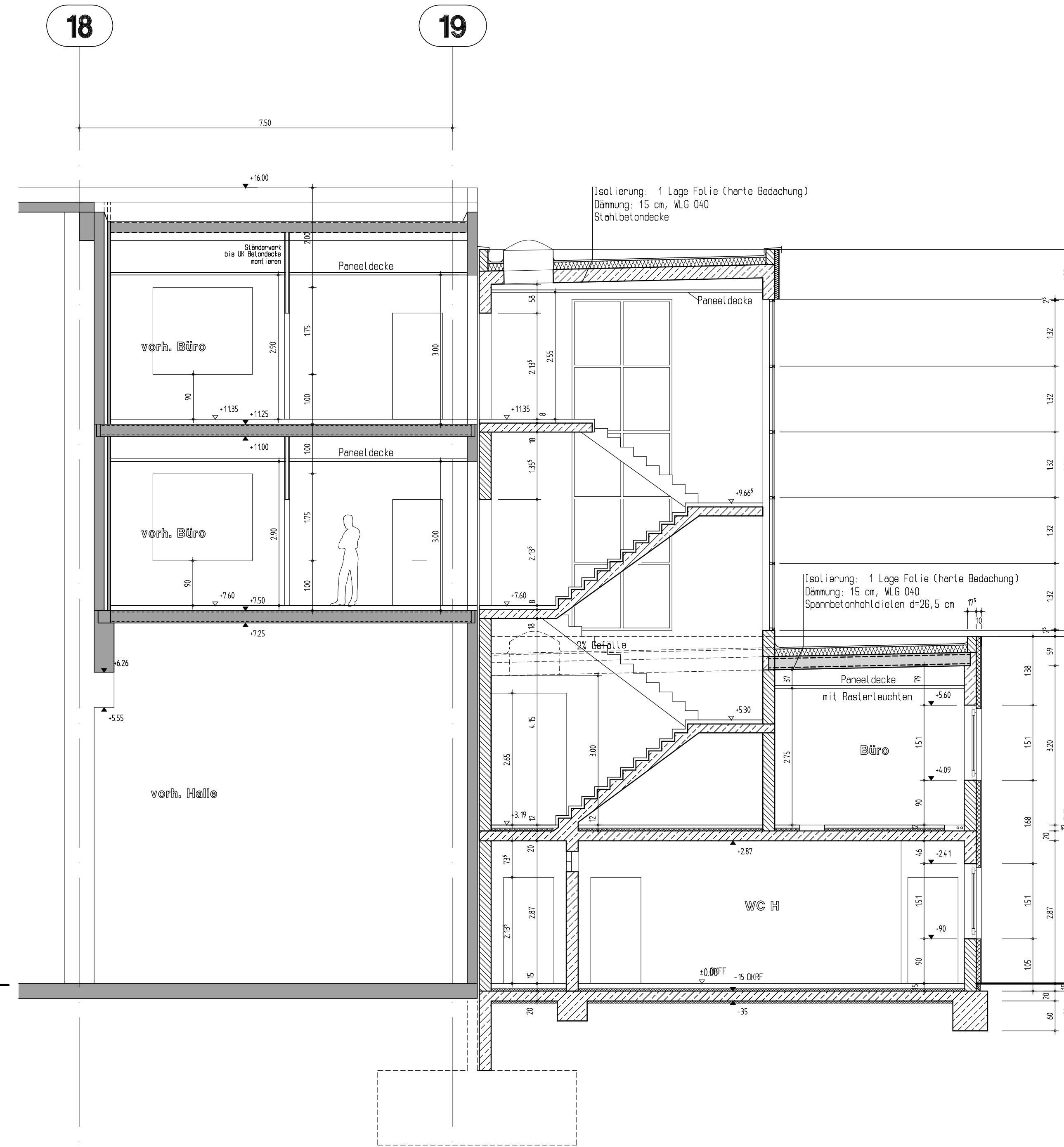
Schnitt 3-3
