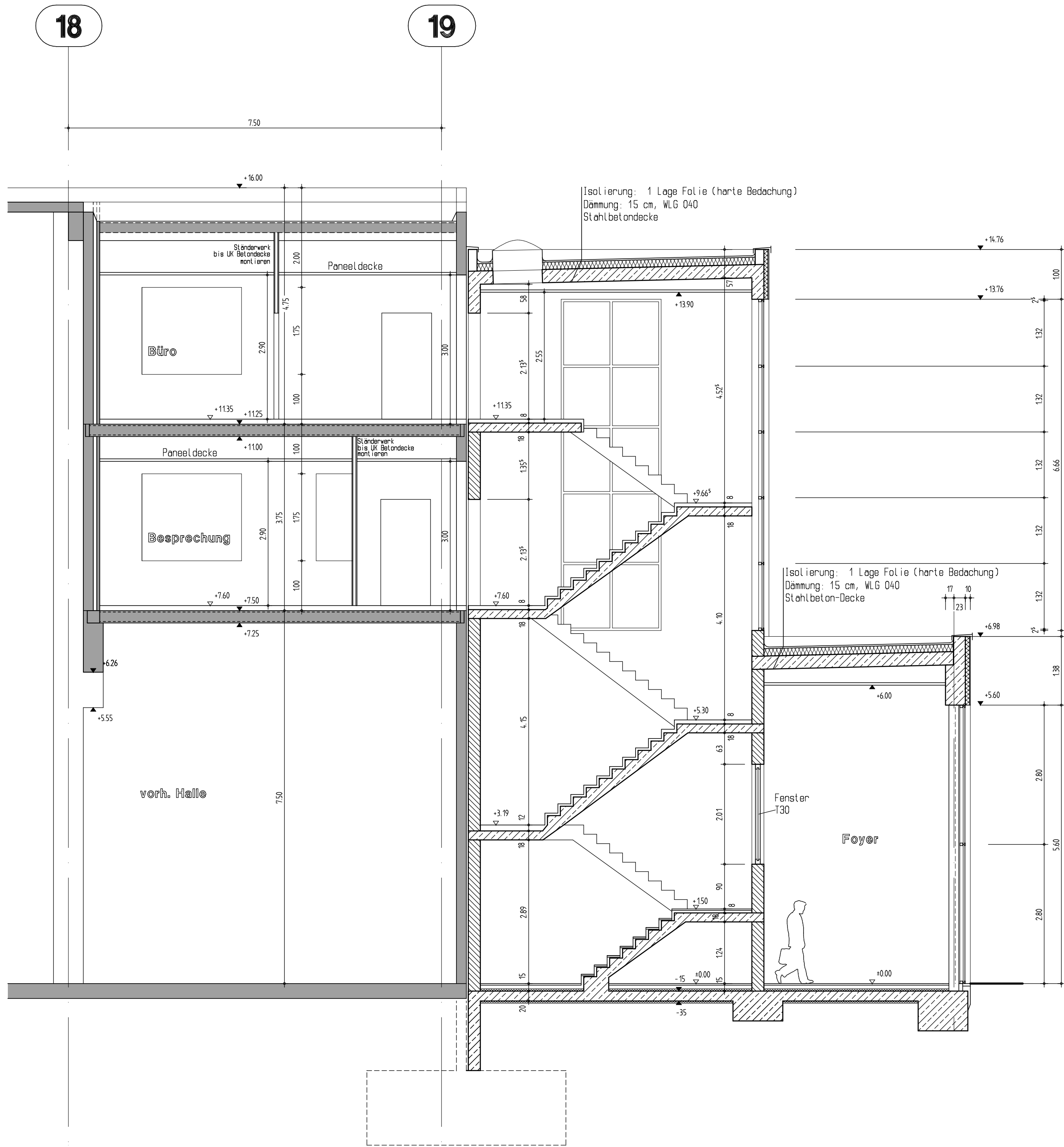
Schnitt 1-1
